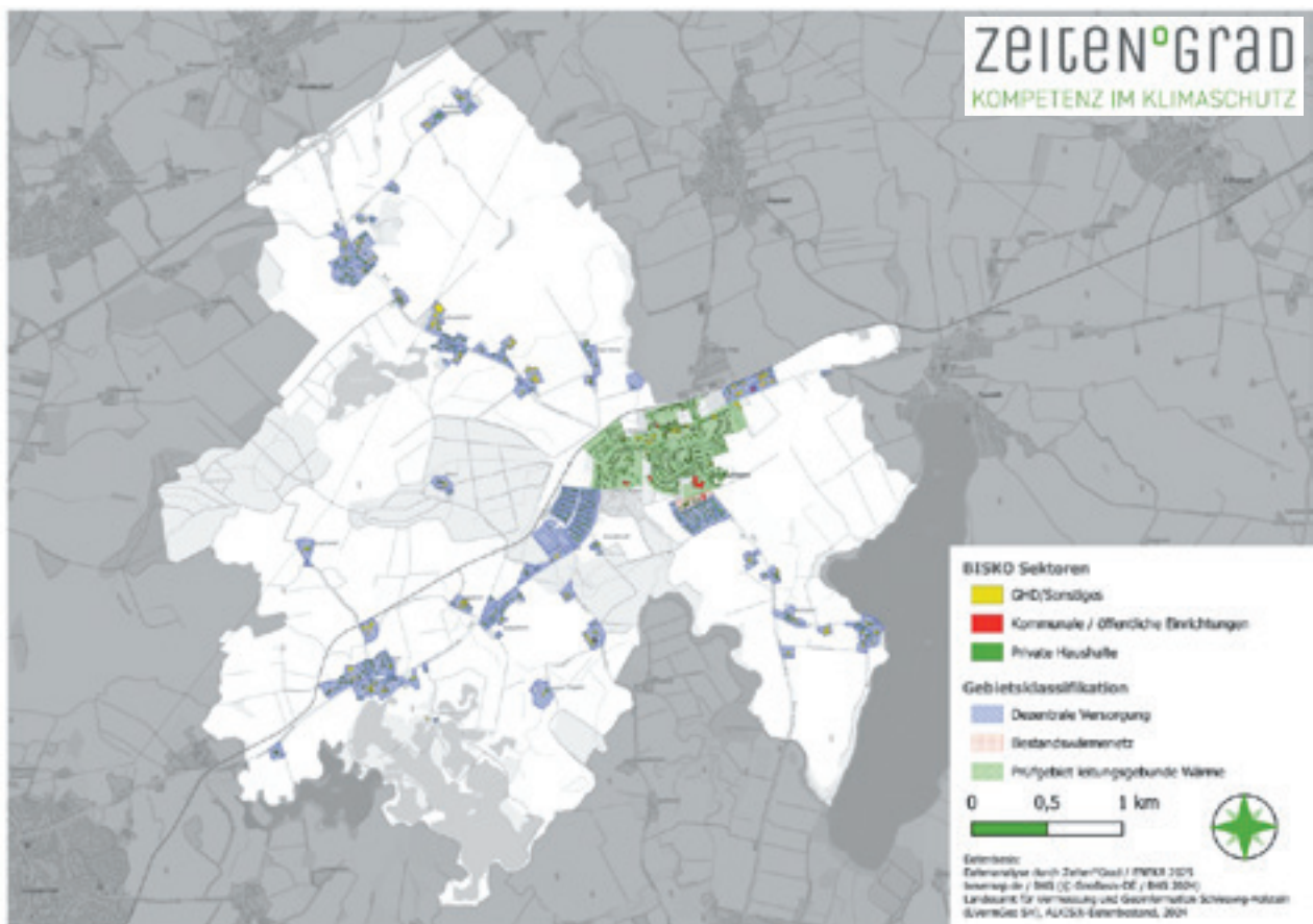
Abbildung 42: Räumliches Konzept zur klimaneutralen Wärmeversorgung der Gemeinde Probsteierhagen als Übersichtskarte. (Quelle: QGIS / LVermGe SH)
